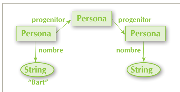
Figura 5. Ejemplo de una consulta de grafo (específicamente de caminos). Considerando el grafo de la Figura 3, la consulta retorna los nombres de los abuelos de "Bart", estos son "Abraham", "Penelope", "Clarcy" y "Jacqueline".
