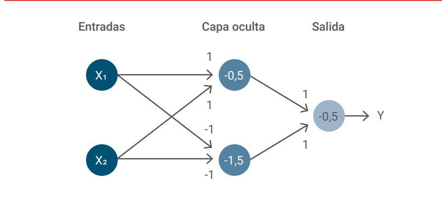
Figura 1. Red neuronal que simula al operador booleano XOR.
