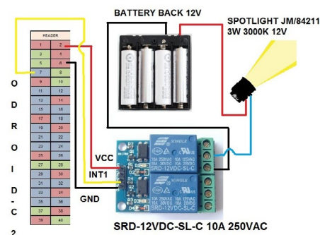
Figura 1 - Diagrama por bloques
