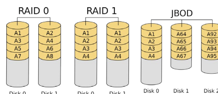
Figura 4 - RAID 0, RAID 1 y JBOD
