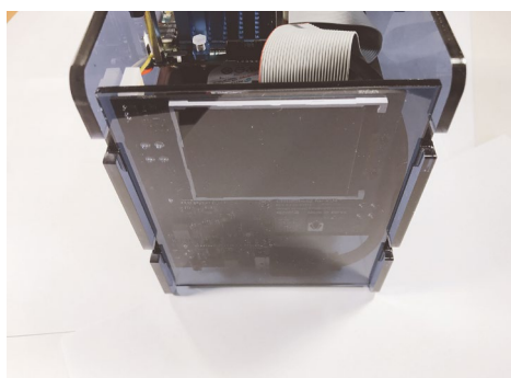
Figura 13 - Coloca la pieza delantera en la parte frontal (C)
