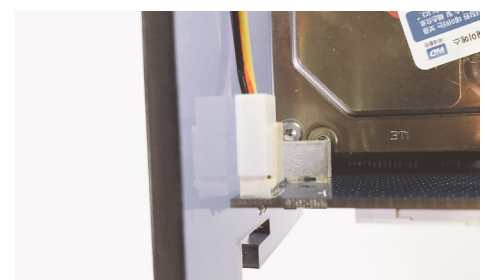
Figura 10 - Inserta el cable del ventilador en la placa CloudShell-2
