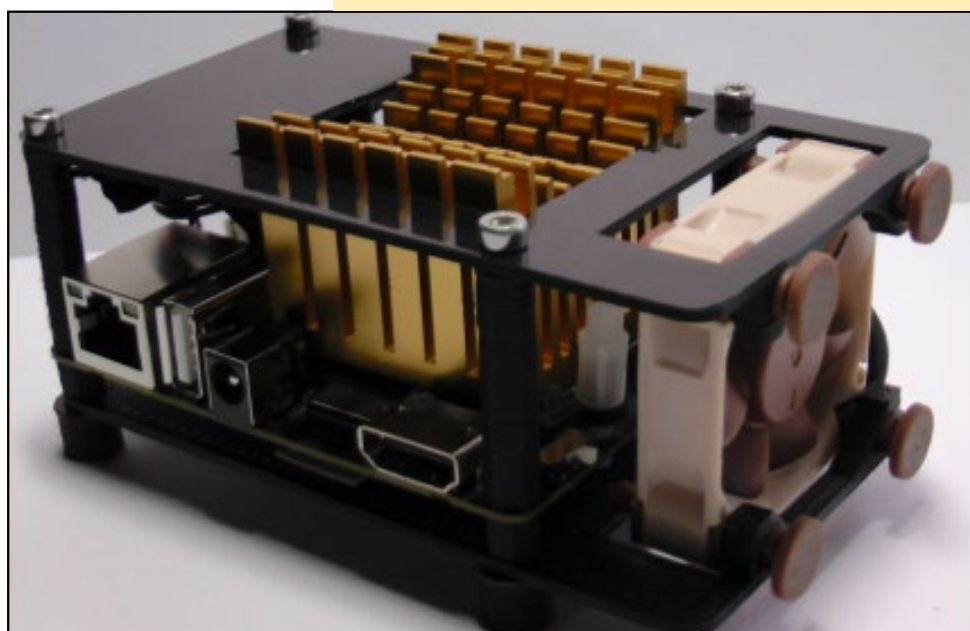
Primer plano del ventilador, puerto HDMI y Ethernet
