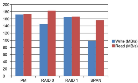
Figura 18 - Rendimiento lectura/escritura de E/S en cada modo de almacenamiento en los 2xHDD WD Red de 6TB
