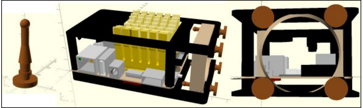
Diseño conceptual de OpenSCAD
