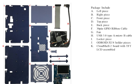
Figura 5 - Piezas incluidas en el kit Cloudshell-2
