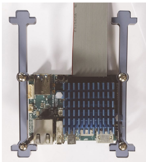
Figura 11 - Monta el ODR0ID-XU4 y las piezas del soporte para XU4 (J + L + M)
