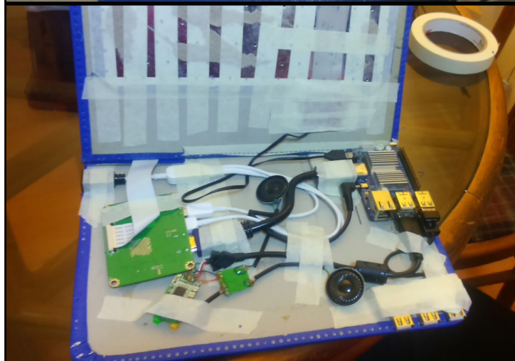
Mirando de cerca el Wawa y a sus componentes internos
