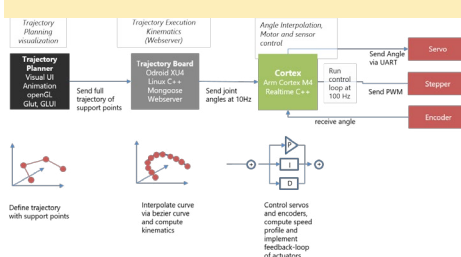
Figura 2 - Flujo de datos de la pila completa
