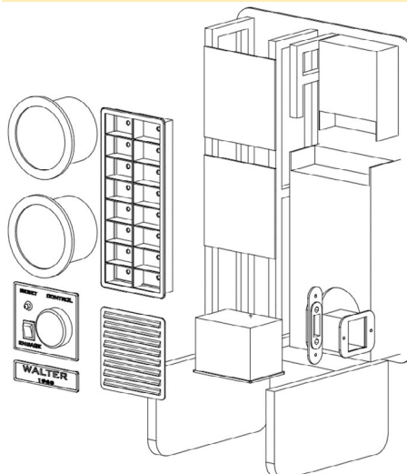
Figura 6 - Desglose de la caja de control
