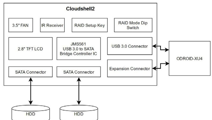
Figura 2 - Diagrama por bloques del CloudShell-2
