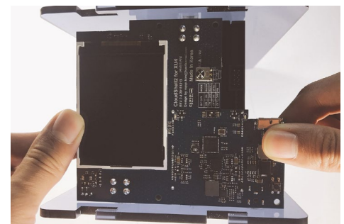
Figura 7 - Conecta la placa CloudShell-2 a los discos duros (K)
