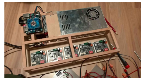
Figura 8 - Interior de la caja
