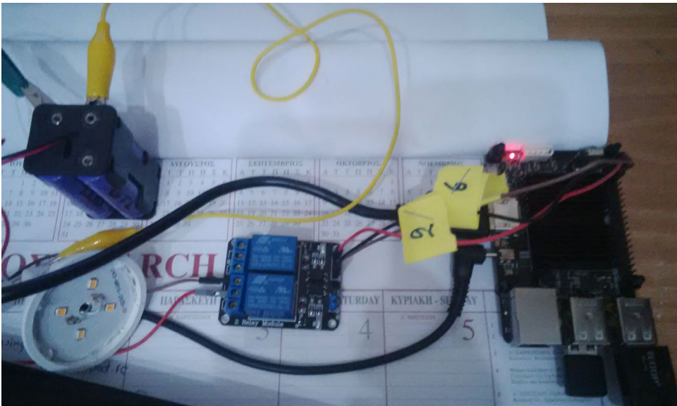
Figura 5 - Configuración del hardware
